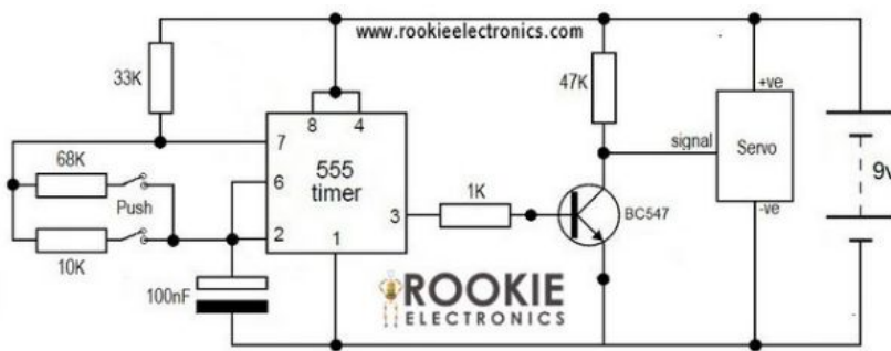
Servotester Bild 1 (68K Widerstand durch 100K Poti ersetzt)
